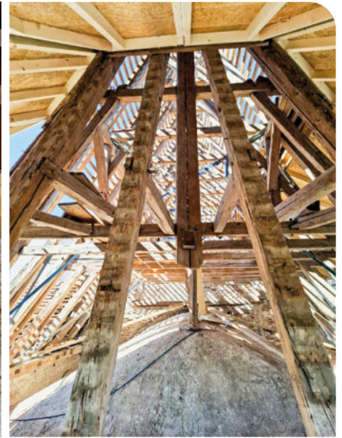
Der Dachstuhl über dem Chor (C. Zieglertrum)
