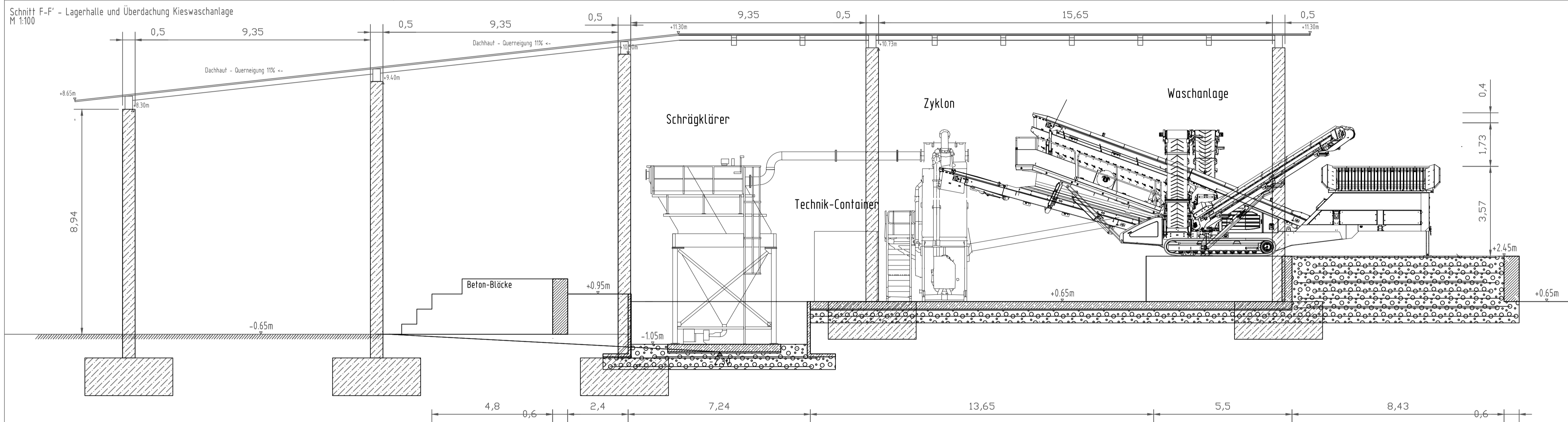
Schnitt I-I' - Lagerhalle für Recyclingmaterial und Bodenaushub M 1:100
