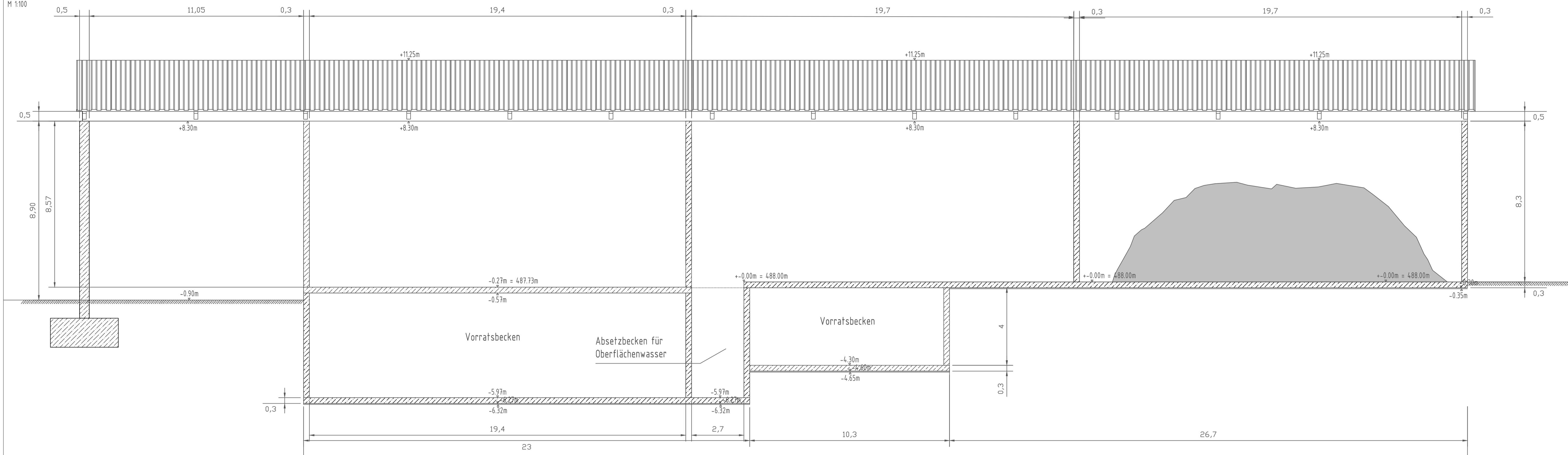
Schnitt F-F' - Lagerhalle und Überdachung Kieswaschanlage M 1:100
